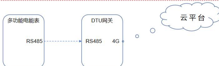
新增设备通信回路示意图
